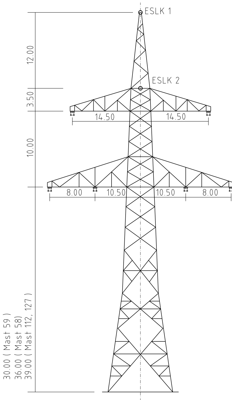
Mast Nr. 58, 59, 112, 127
